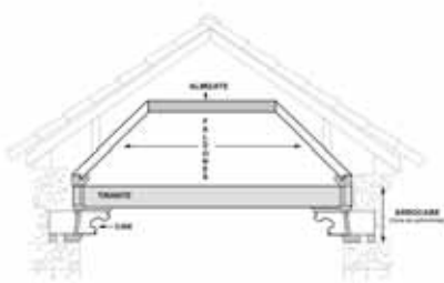
Esquema de corte en sección.
